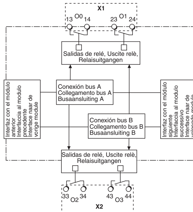
Fig. 1: Schema connessioni
